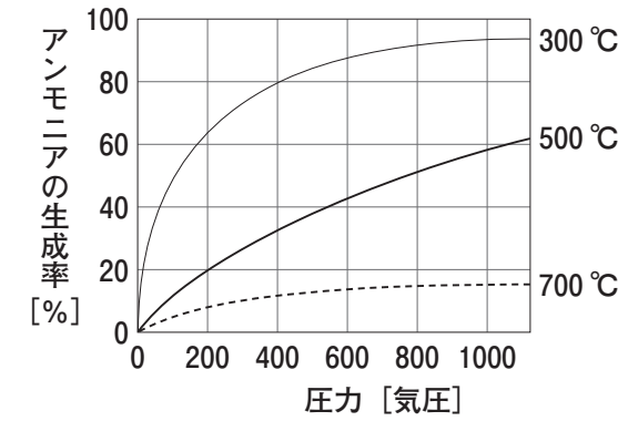
図3 アンモニアの生成率と圧力の関係
