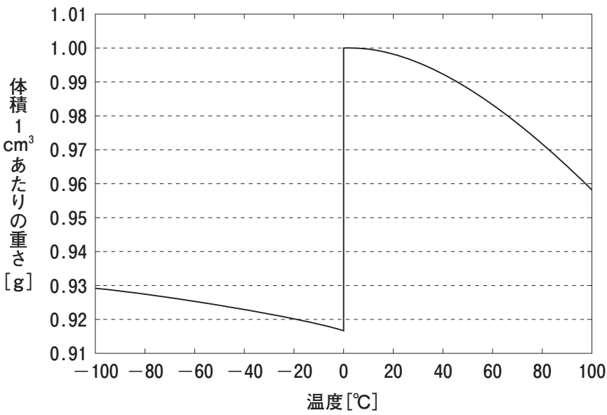
図2 水、氷1cm 3 あたりの重さと温度の関係
